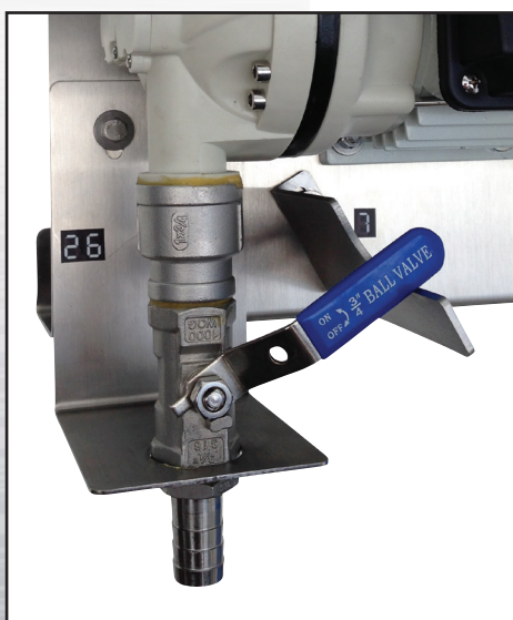
Hefboom rechts tegen aanslag, 8 Ltr. / Min.
